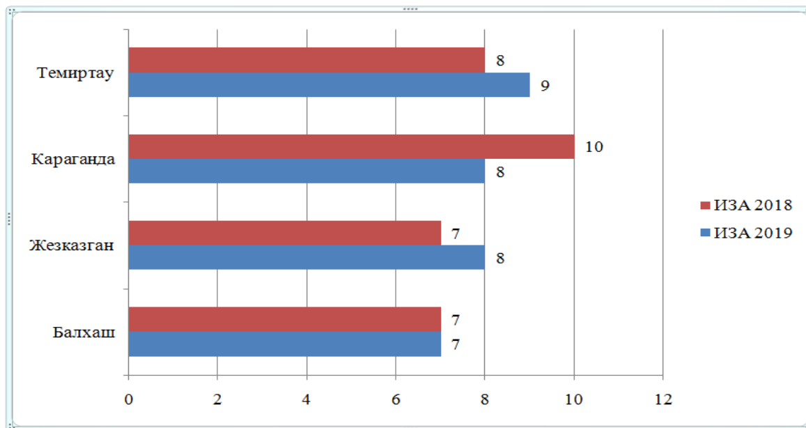
Рисунок 2 – Уровень загрязнения населенных пунктов Карагандинской области (ИЗА 2018 и ИЗА 2019 года)
