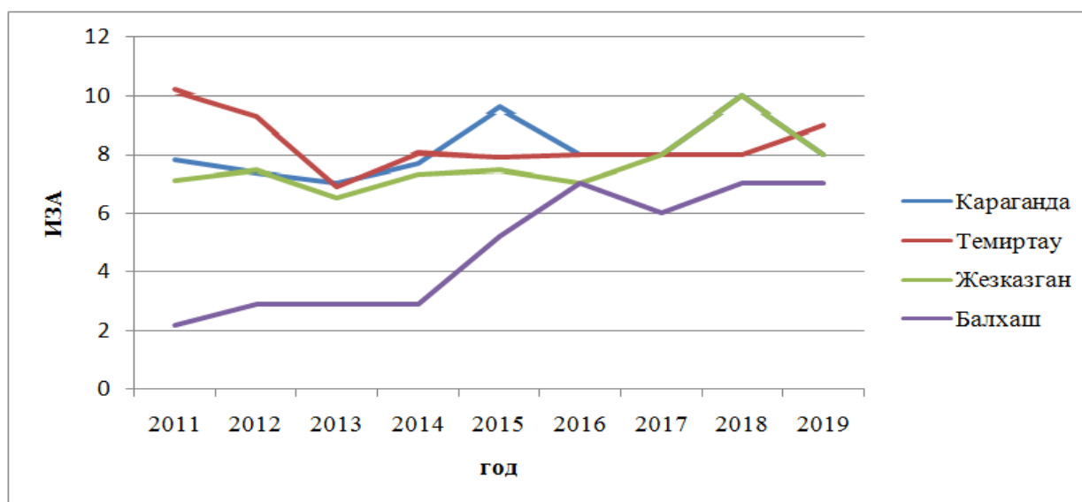
Рисунок 3 – Уровень загрязнения населенных пунктов промышленных центров Карагандинской области (ИЗА 2011- 2019 гг.)
