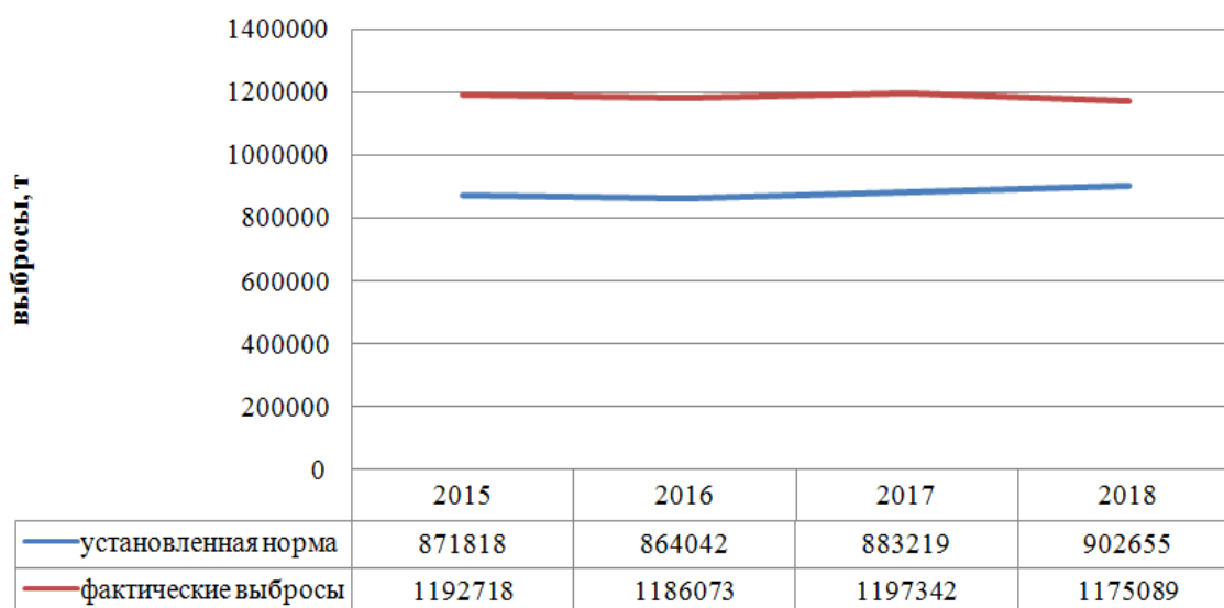
Рисунок 1 – Динамика атмосферных выбросов (в тыс. тонн) в Карагандинской области за 2015-2018 гг.
